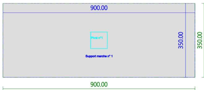
Développé intérieur vu de dessous Support marche n° 1 à 10
